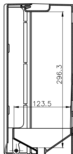
A-A断面図
