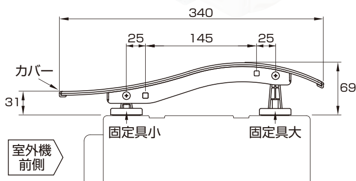
寸法図(mm)
