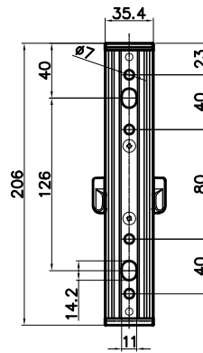
壁付金具詳細図 Scale/1:5
