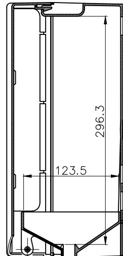
A-A断面図
